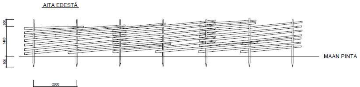
Periaatekuva riukuaidan toteutuksesta © Viherteema Oy
